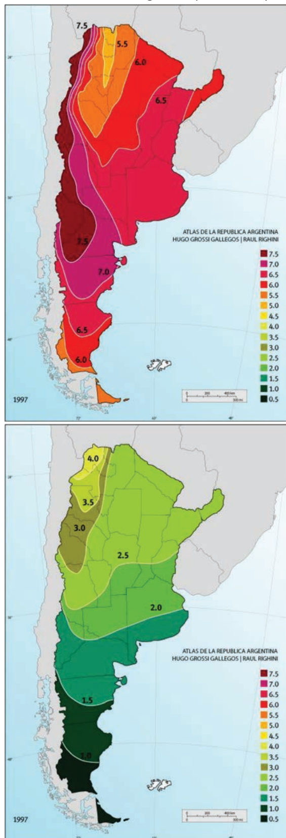
Figura 25. Mapas de radiación solar en Argentina en enero (arriba) y julio (abajo) en kWh/m². Fuente: Atlas de Energía Solar de Argentina Continuará...
