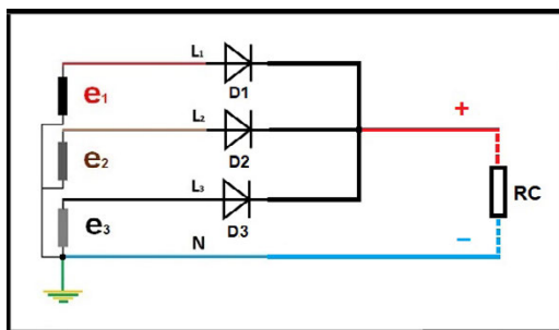
Figura 1 - Esquema de conexiones de una fuente trifásica de media onda
