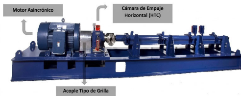
Figura 1. Sistema de bombeo horizontal (Hpump).
